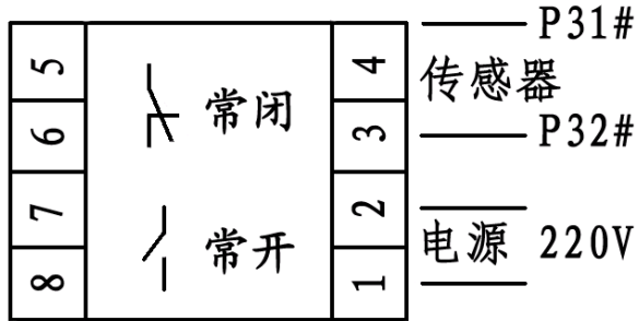
LB05/LB10-II 接线图
