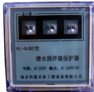
正面外观图
