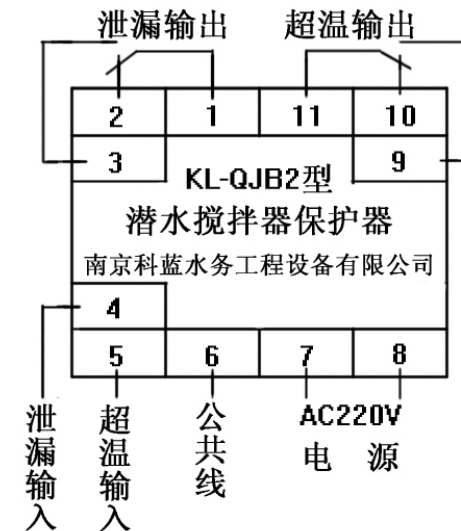
接线端子图
